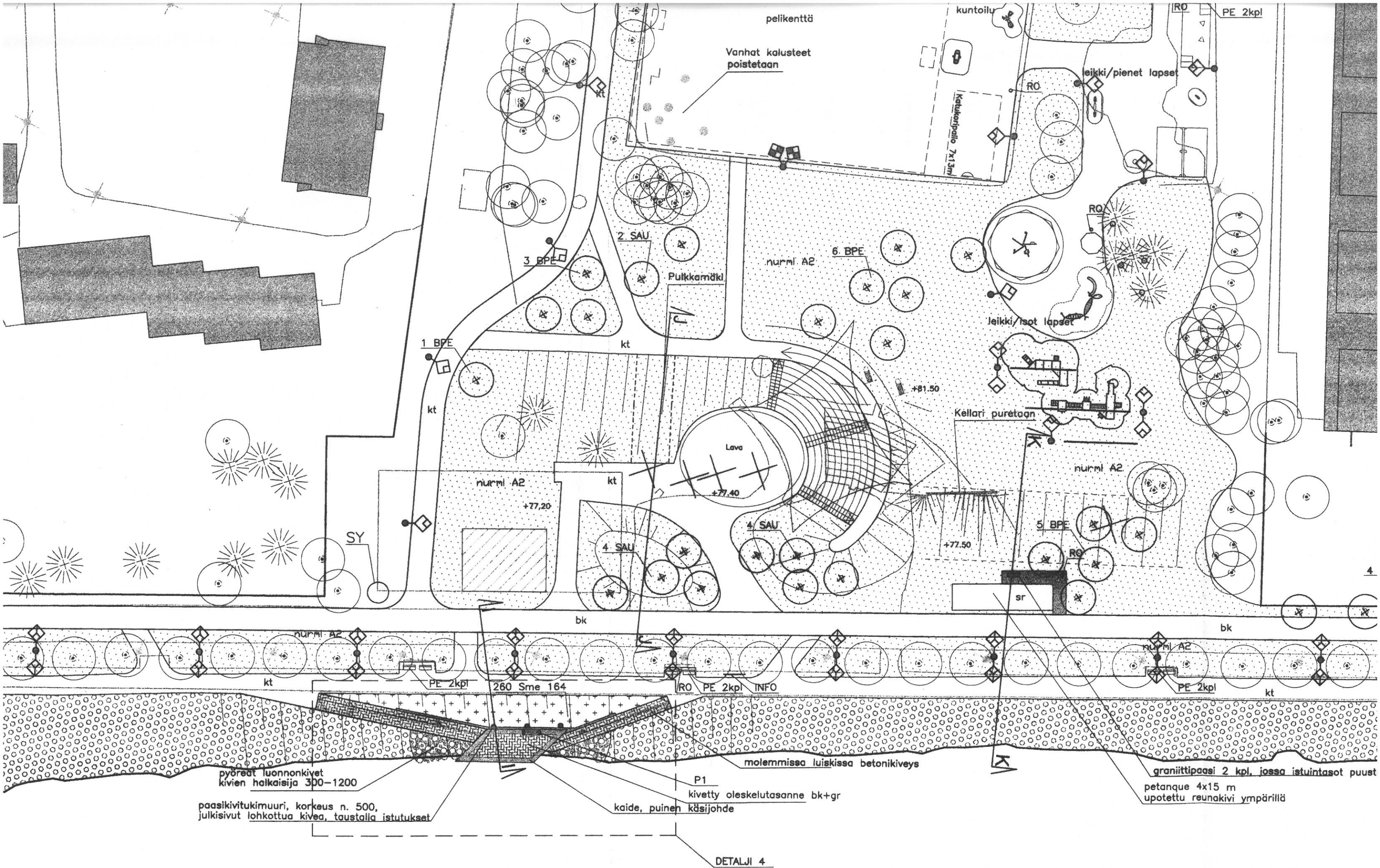
Konttisenpuisto, ympäristösuunnitelma; ote piirustuksesta no 7257A-272
